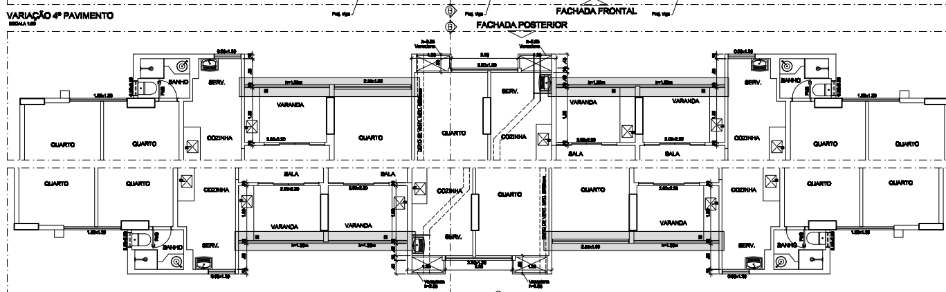
VARIAÇÃO 13º ao 18º PAVIMENTO MEDIDA 1:50
